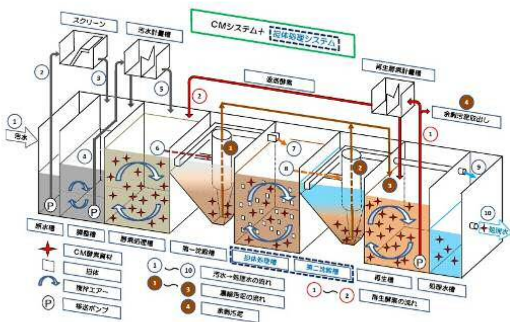
排水処理システムフロー図
